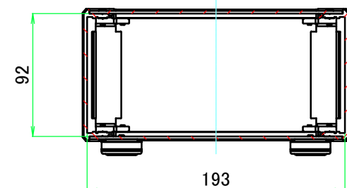
A-A (1:4)
