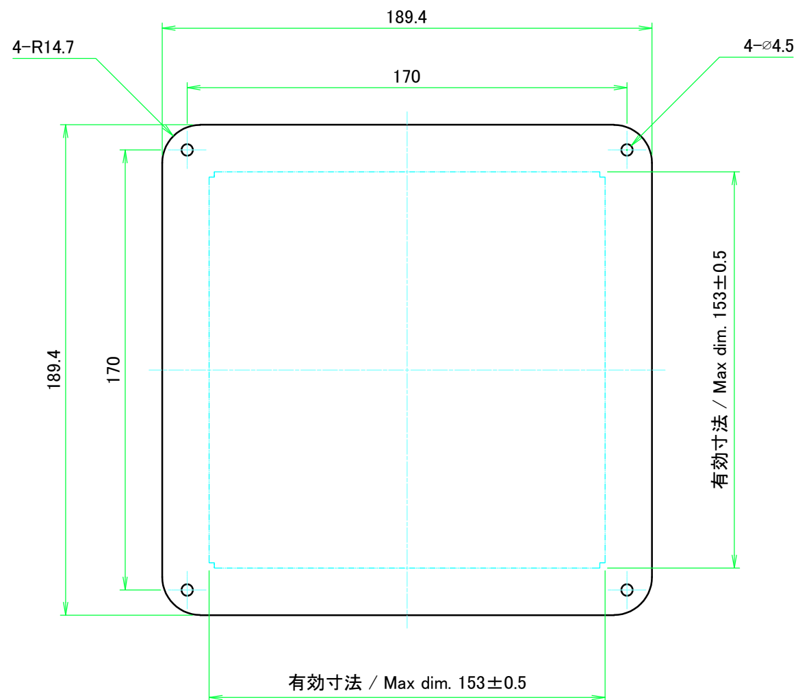
保護シート側 Surface protective film side
