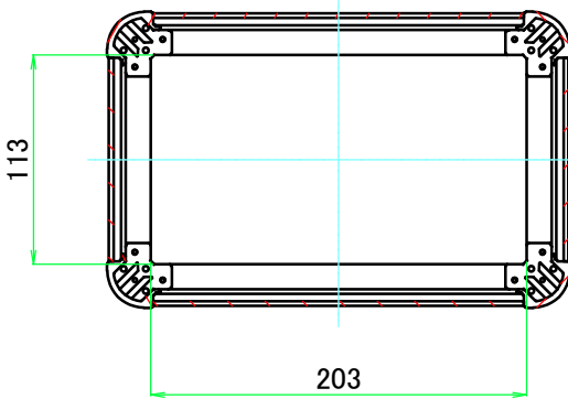
C-C ( 1 : 4.5 )
