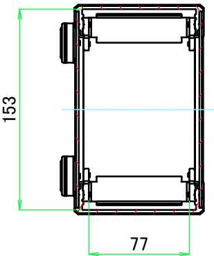
B-B ( 1 : 4 )
