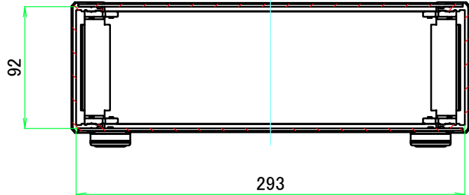
A-A ( 1 : 4 )
