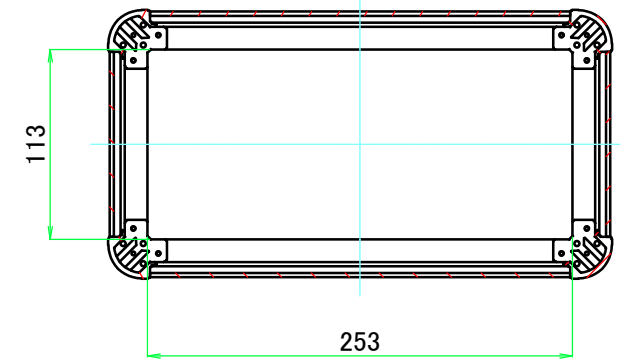
C-C ( 1 : 4.5 )
