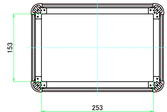
C-C ( 1 : 4.5 )
