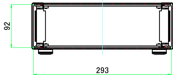
A-A ( 1 : 5 )
