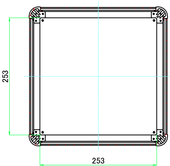
C-C ( 1 : 5 )
