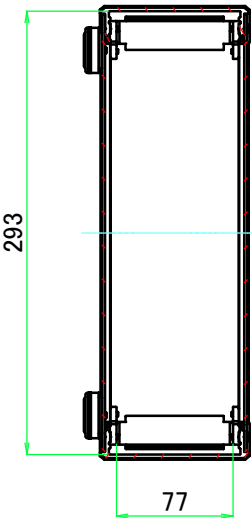
B-B ( 1 : 5 )
