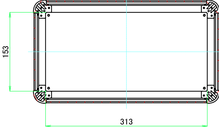
C-C ( 1 : 4.5 )
