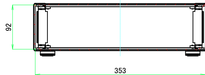
A-A ( 1 : 4.5 )
