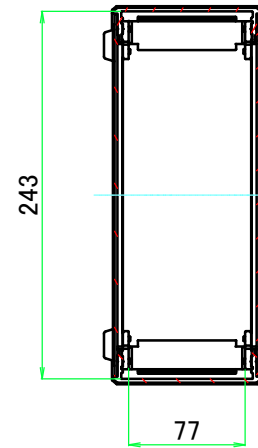
A-A (1:5)
