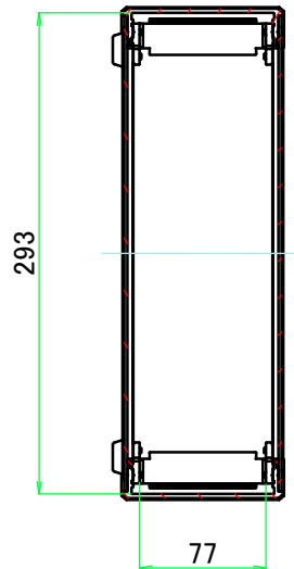
A-A (1:5)
