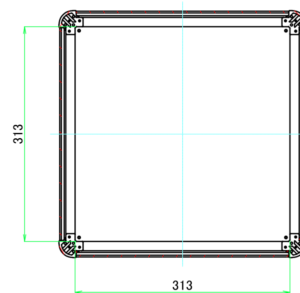
C-C ( 1 : 5.5 )
