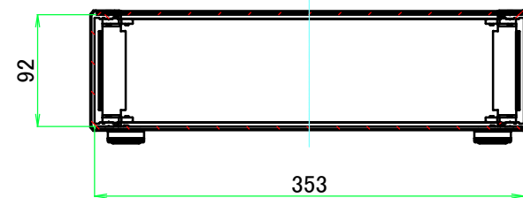
A-A ( 1 : 5.5 )
