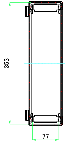
B-B ( 1 : 5.5 )
