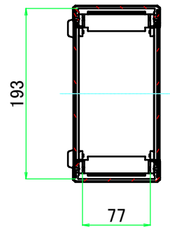
A-A (1:6)
