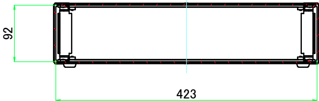
B-B ( 1 : 6 )
