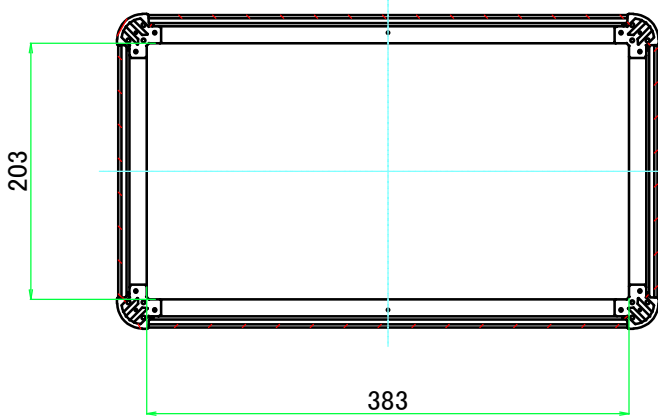
C-C ( 1 : 6 )
