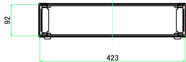
B-B ( 1 : 6.5 )
