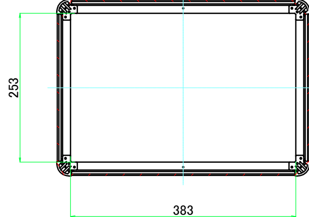
C-C ( 1 : 6.5 )
