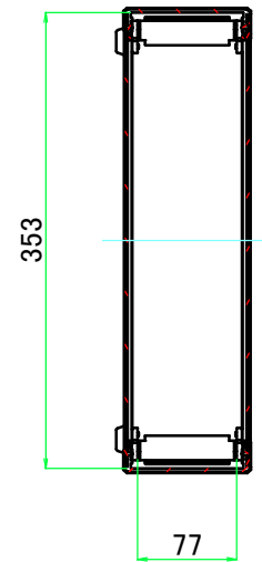
A-A ( 1 : 6.5 )
