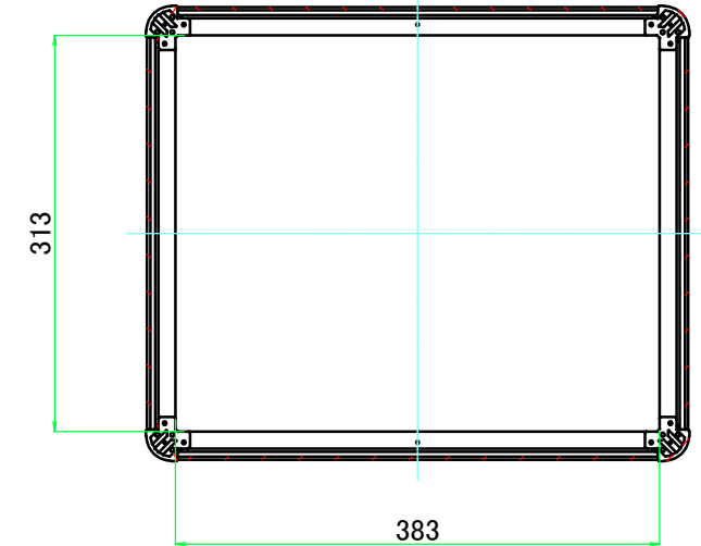
C-C ( 1 : 6.5 )
