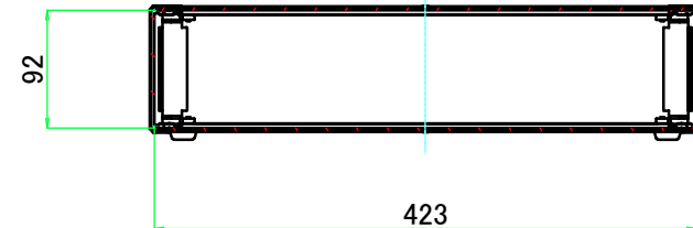
B-B ( 1 : 6.5 )
