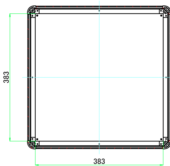
C-C ( 1 : 6.5 )
