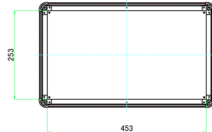
C-C ( 1 : 6.5 )
