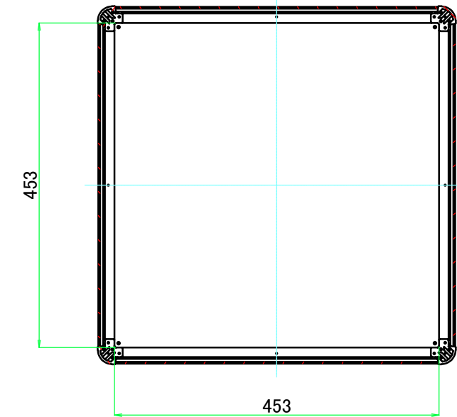
C-C ( 1 : 7.5 )
