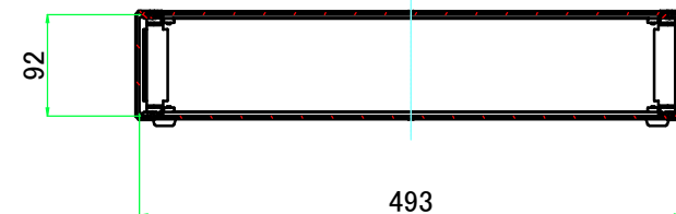
B-B ( 1 : 7.5 )
