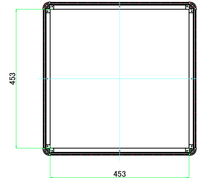
C-C ( 1 : 7.5 )
