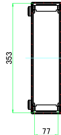
B-B ( 1 : 7.5 )
