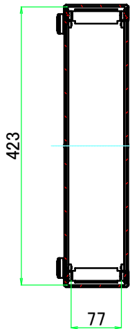
B-B ( 1 : 8 )
