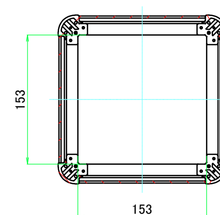
C-C ( 1 : 4.5 )
