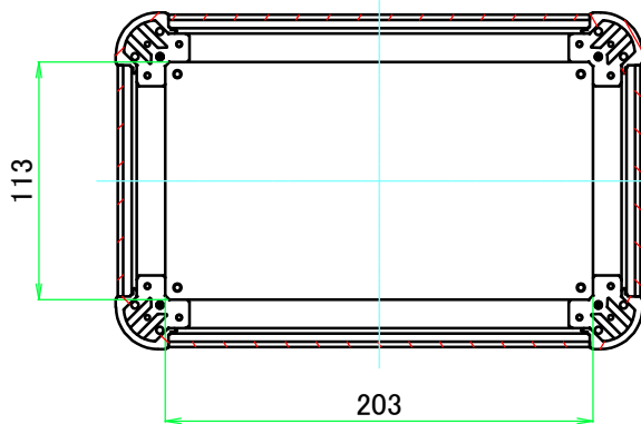
C-C ( 1 : 4 )
