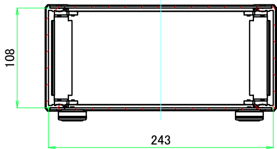
B-B ( 1 : 4 )
