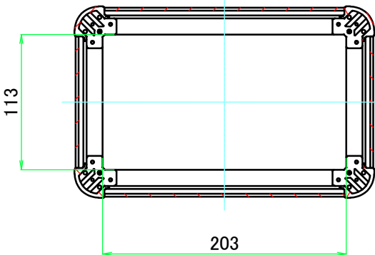
C-C ( 1 : 4.5 )
