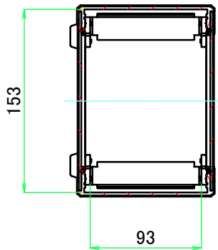
A-A ( 1 : 4.5 )
