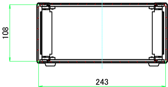
B-B ( 1 : 4.5 )
