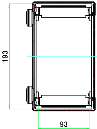
A-A (1:4)
