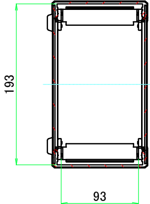
A-A ( 1 : 4.5 )
