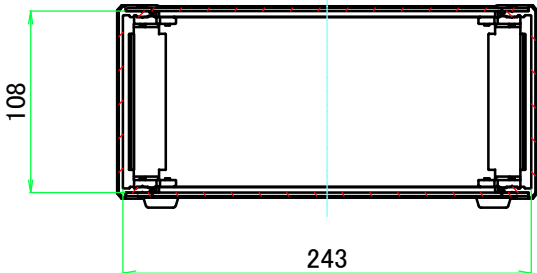
B-B ( 1 : 4.5 )
