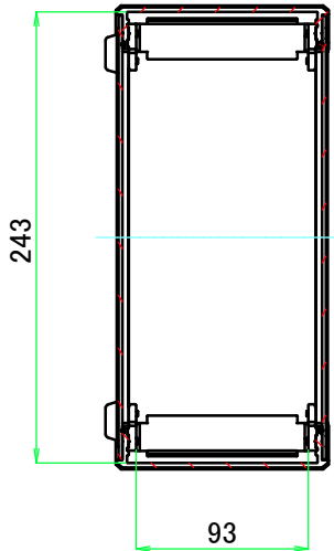
A-A ( 1 : 4.5 )
