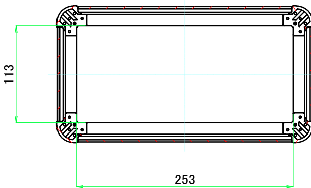
C-C ( 1 : 4.5 )
