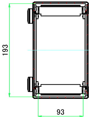
A-A ( 1 : 4.5 )
