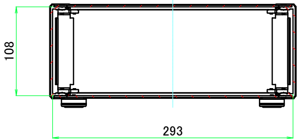
B-B ( 1 : 4.5 )
