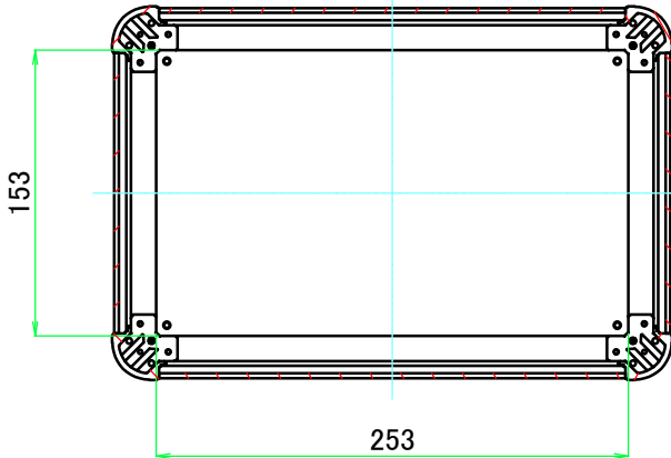
C-C ( 1 : 4.5 )
