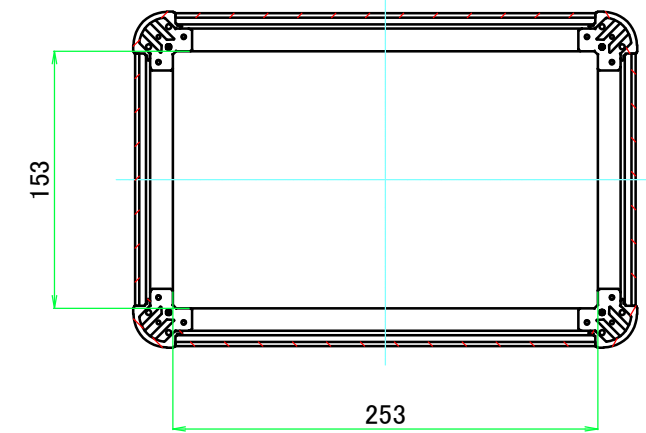
C-C ( 1 : 4.5 )
