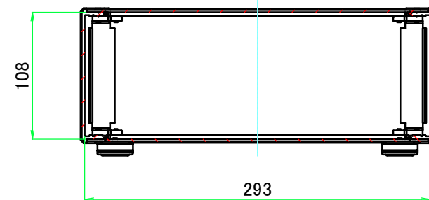
B-B ( 1 : 4.5 )
