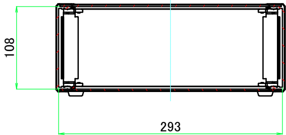
B-B ( 1 : 5 )
