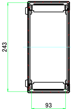
A-A ( 1 : 5 )
