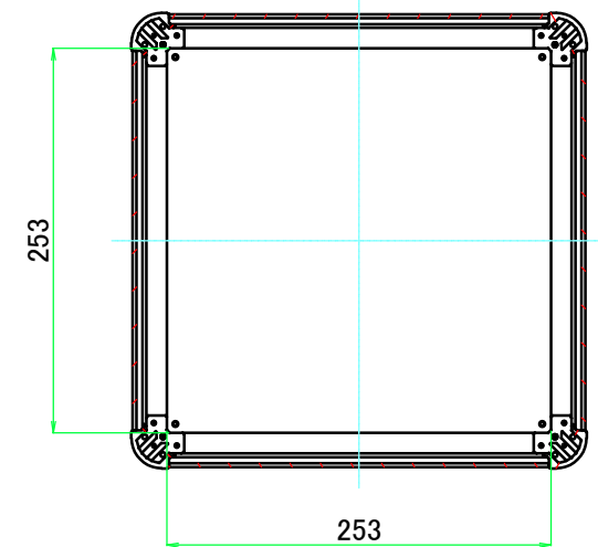
C-C ( 1 : 5.5 )
