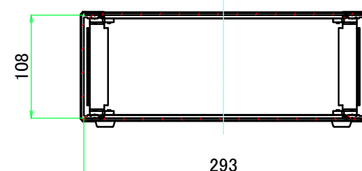
B-B ( 1 : 5.5 )
