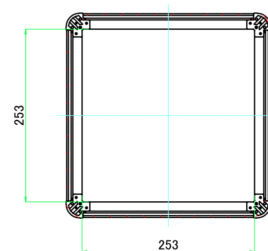
C-C ( 1 : 5.5 )
