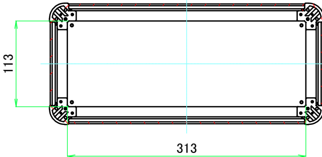
C-C ( 1 : 5 )
