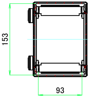
A-A ( 1 : 5 )
