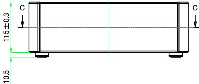
B-B ( 1 : 5 )
