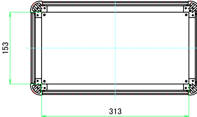
C-C ( 1 : 5 )
