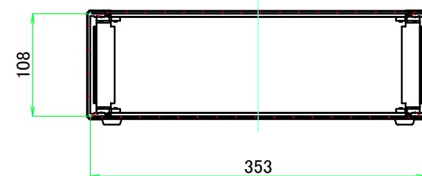
B-B ( 1 : 5.5 )
