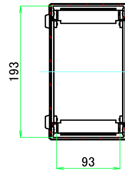
A-A ( 1 : 5.5 )
