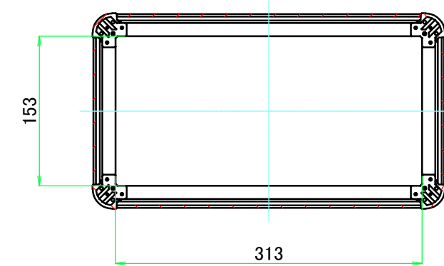
C-C ( 1 : 5.5 )
