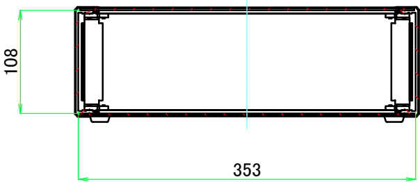
B-B ( 1 : 5.5 )
