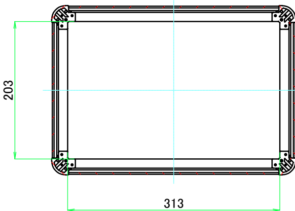
C-C ( 1 : 5.5 )
