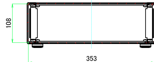
B-B ( 1 : 5.5 )
