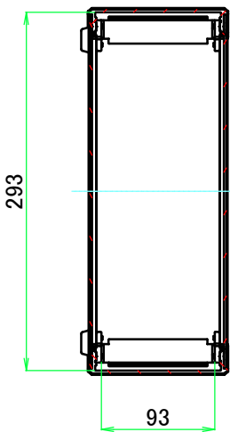
A-A ( 1 : 5.5 )
