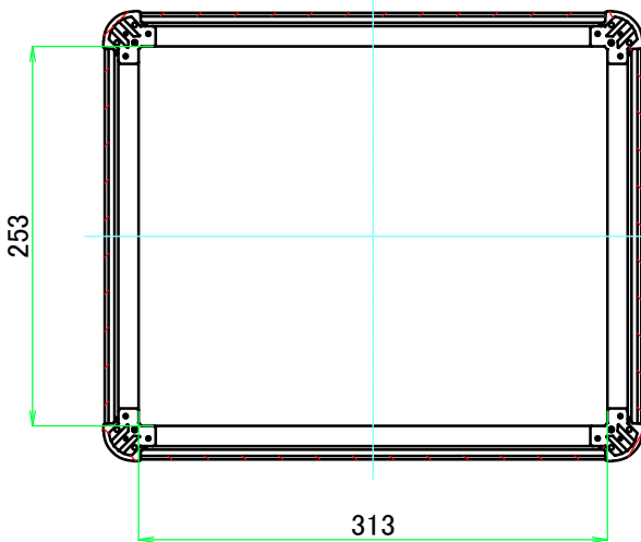
C-C ( 1 : 5.5 )
