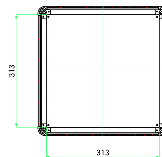
C-C ( 1 : 6.5 )
