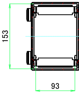
A-A ( 1 : 5.5 )
