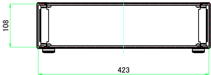
B-B ( 1 : 5.5 )
