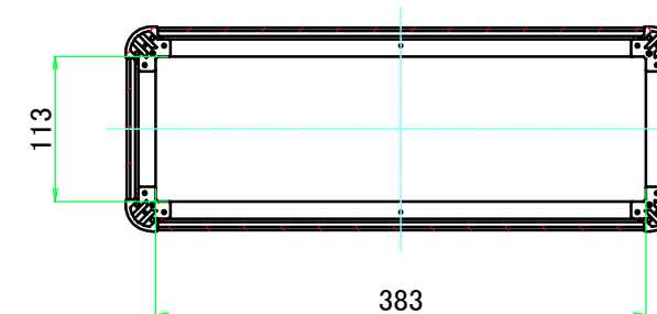
C-C ( 1 : 6.5 )
