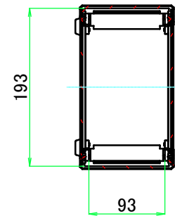
A-A ( 1 : 6.5 )
