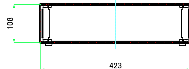
B-B ( 1 : 6.5 )
