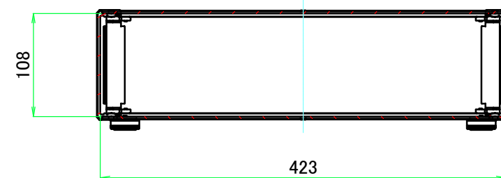
B-B ( 1 : 5.5 )
