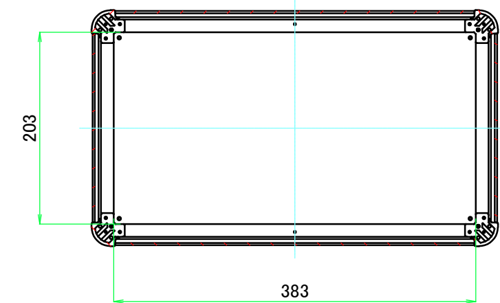
C-C ( 1 : 5.5 )
