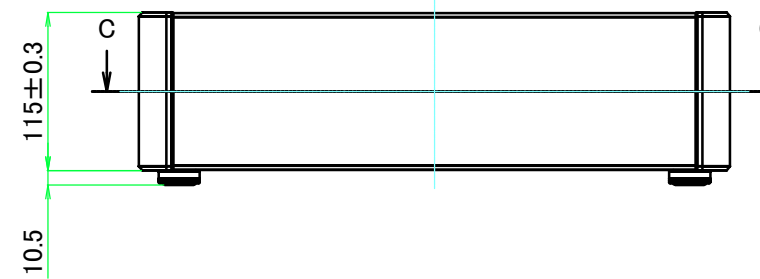
B-B ( 1 : 5.5 )
