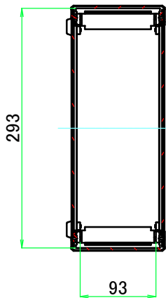
A-A ( 1 : 6.5 )
