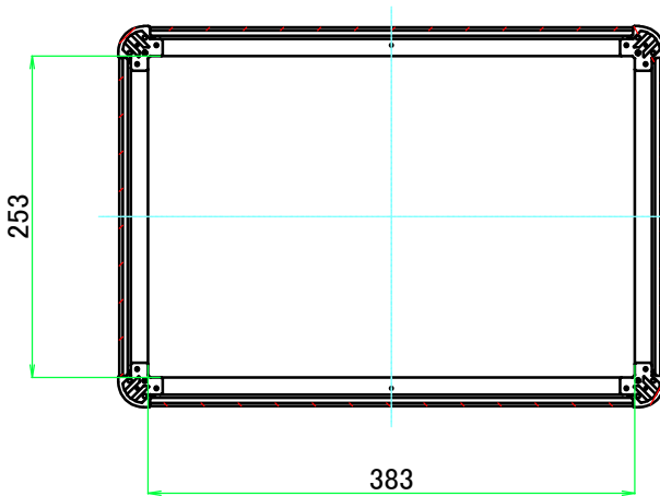
C-C ( 1 : 6.5 )
