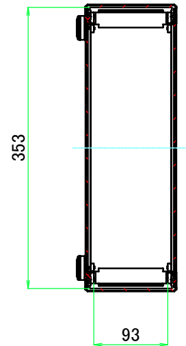
A-A ( 1 : 6.5 )
