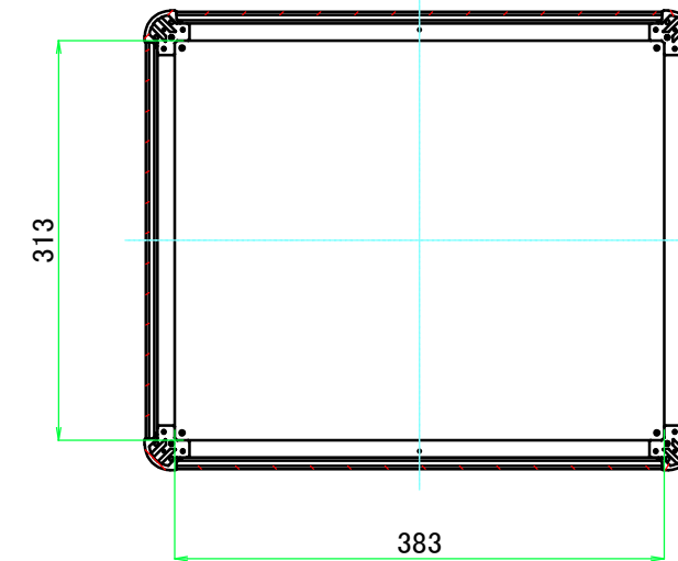
C-C ( 1 : 6.5 )
