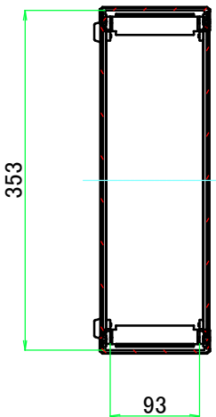
A-A ( 1 : 7 )
