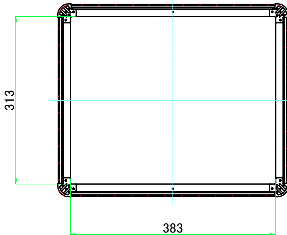
C-C ( 1 : 7 )
