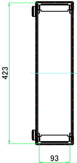
A-A (1:7)
